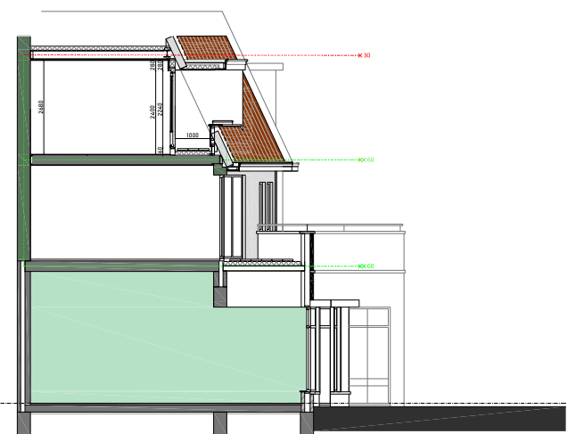
- Doorsnede -
