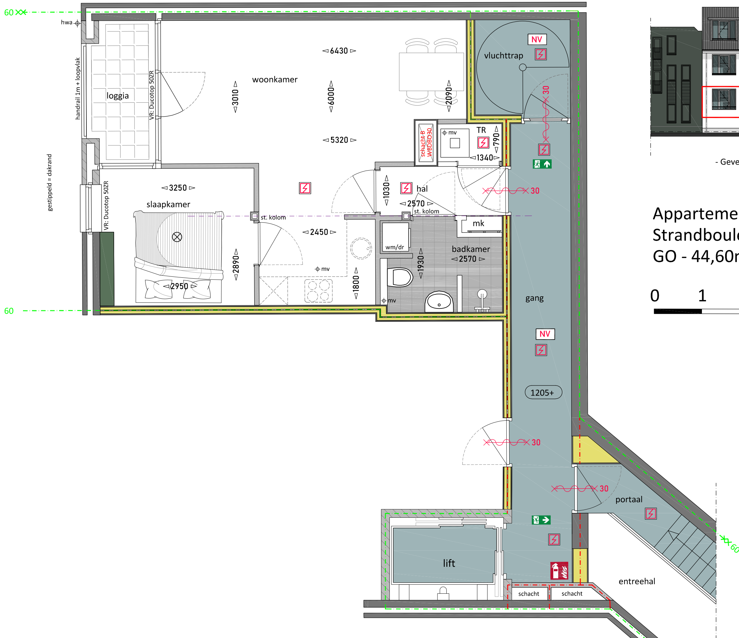
Niveau 1205+ PEIL
